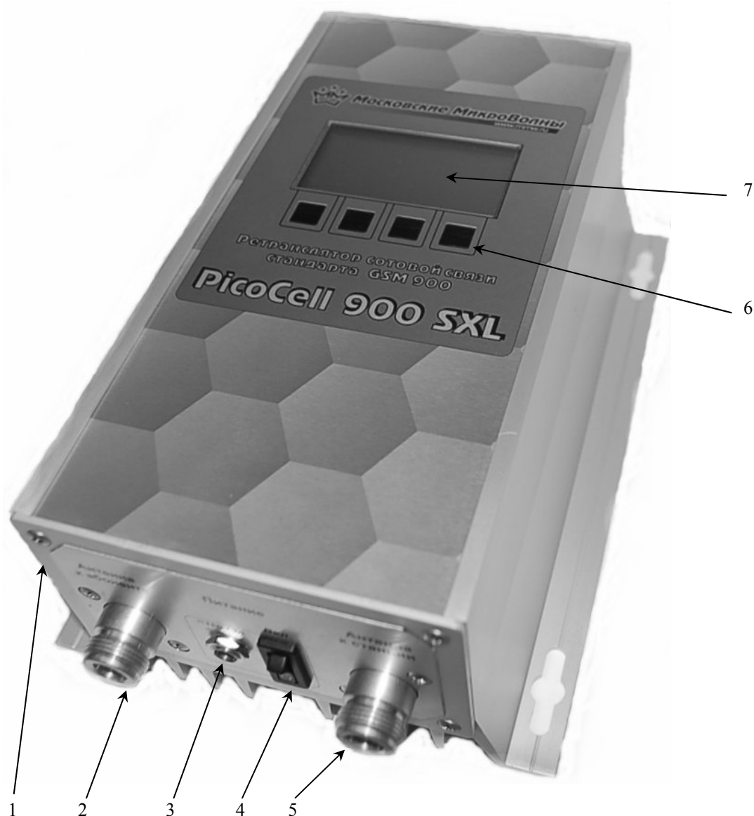
Рис.1 Ретранслятор PicoCell 900 SXL
